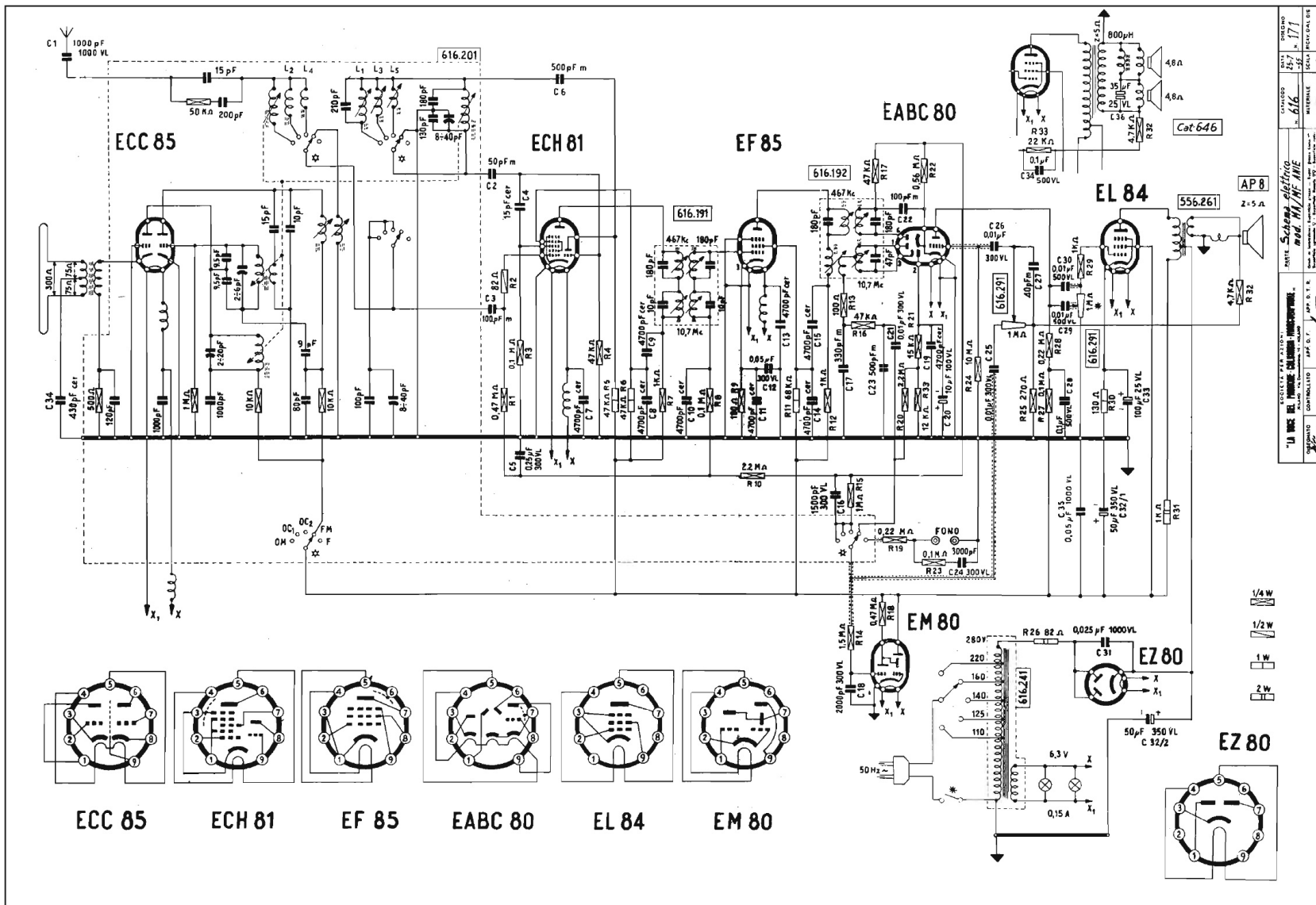
VOCE DEL PADRONE - Modd. AM/FM 616 Anic e 646. Apparecchi a modulazione d'ampiezza e di frequenza, con tre gamme AM e onde medie, corte e cortissime e una banda FM a onde ultracorte. Media frequenza a 465 kc/s e FM a 10,7 Mc/s. Lo schema è del mod. 616; è riportata la differenza per il mod. 646 bifenico. Potenza d'usc. indist. 4 watt. Prod. 1955-56.
